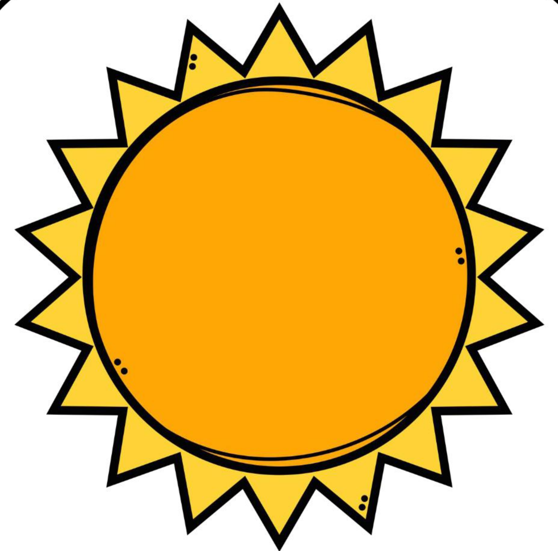
خورشید
