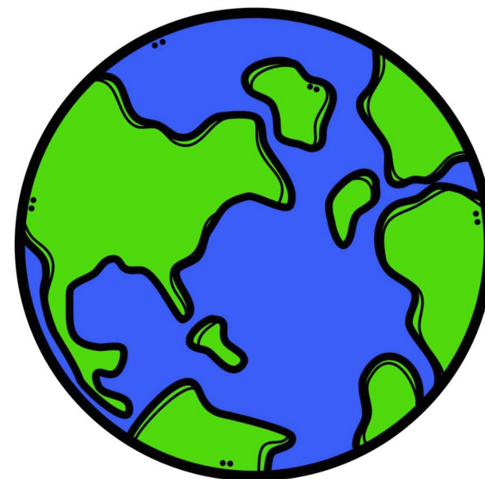
زمین
