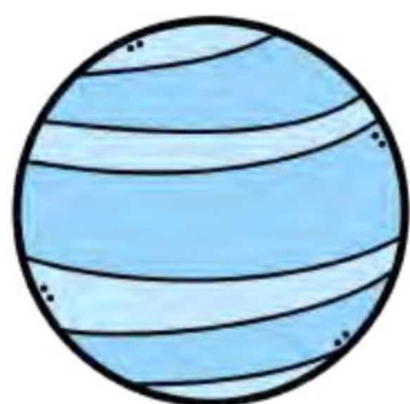
اورانوس
