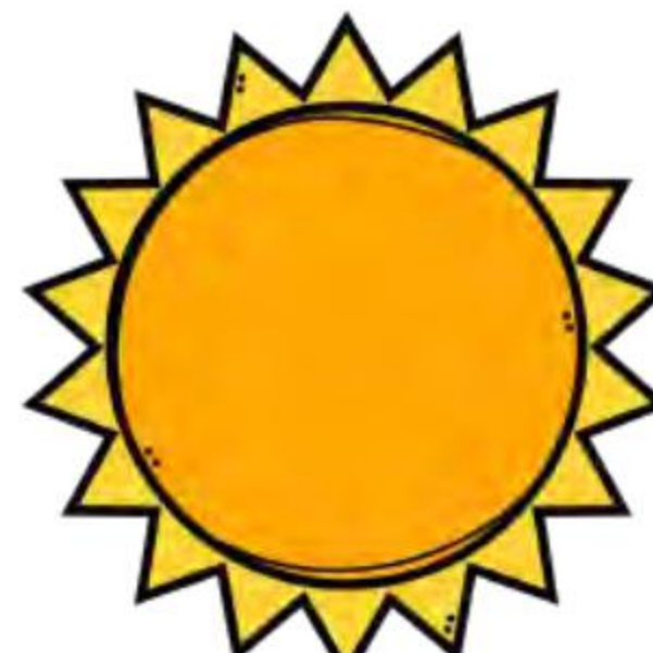
خورشید
